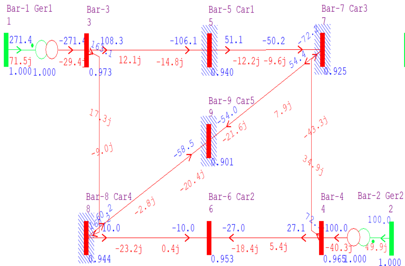
Diagrama no ANAREDE do STB-9 150% na barra 9 sem compensação
