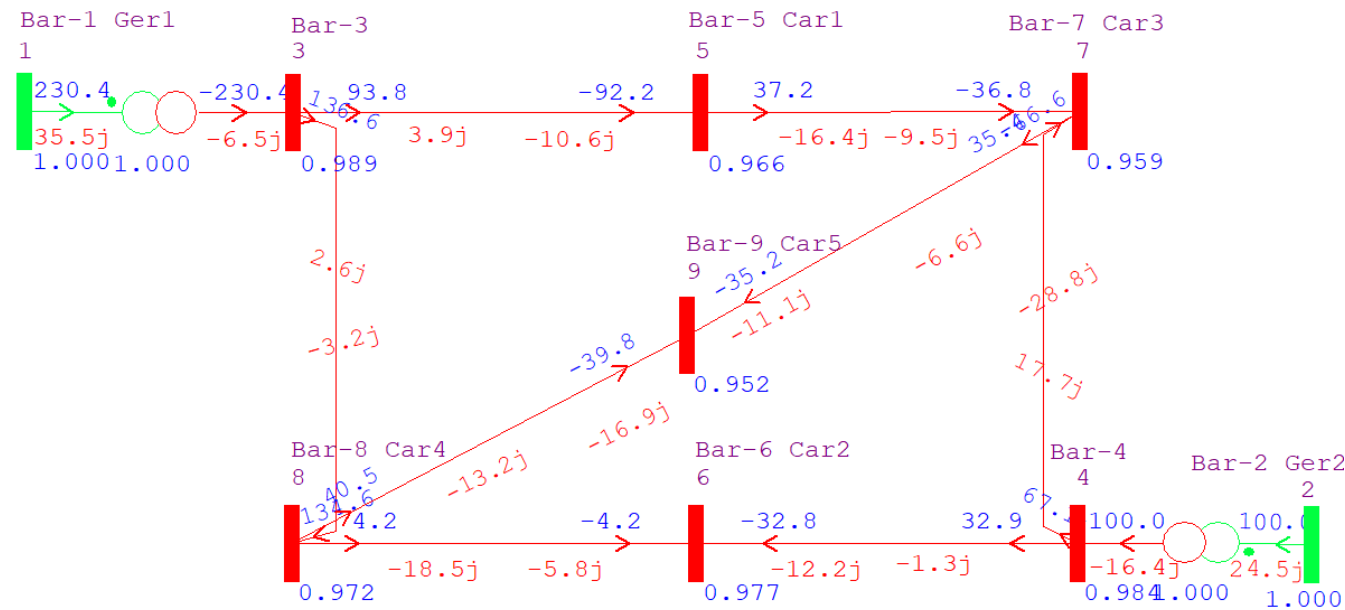
Diagrama no ANAREDE do STB-9 – Caso base
