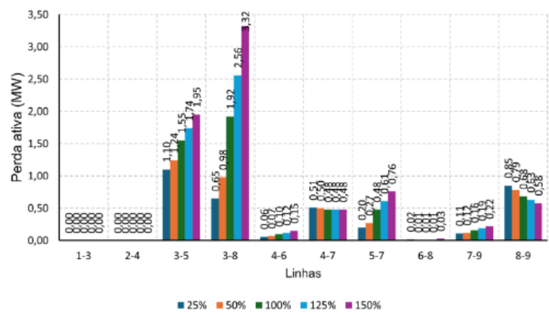
Perdas ativas por linha variação da carga na barra 8.
