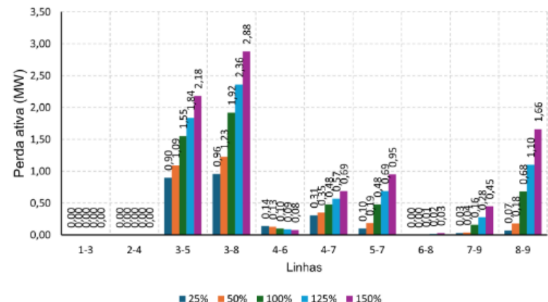
Perdas ativas por linha variação da carga na barra 9.
