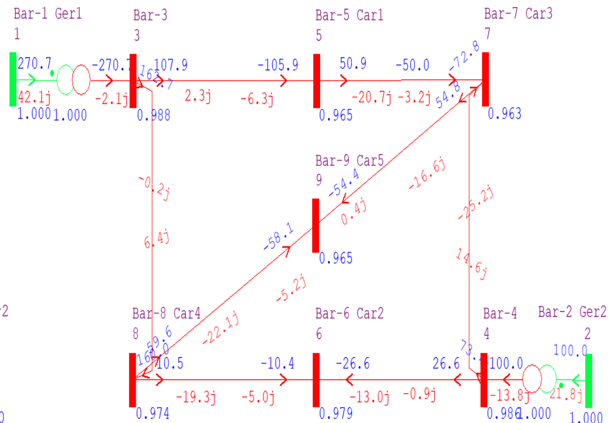
Diagrama no ANAREDE do STB-9 150% na barra 9 com compensação
